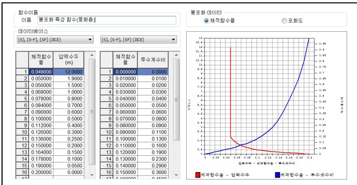
【그림 65.15】 압력수두-체적함수물(포화도)-투수계수비 함수
