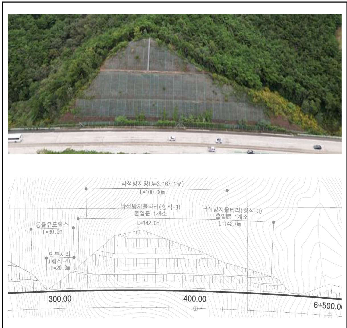
【그림 65.14】 상주절토65 검토대상 비탈면구간
